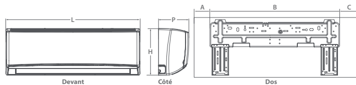
Unité intérieure
