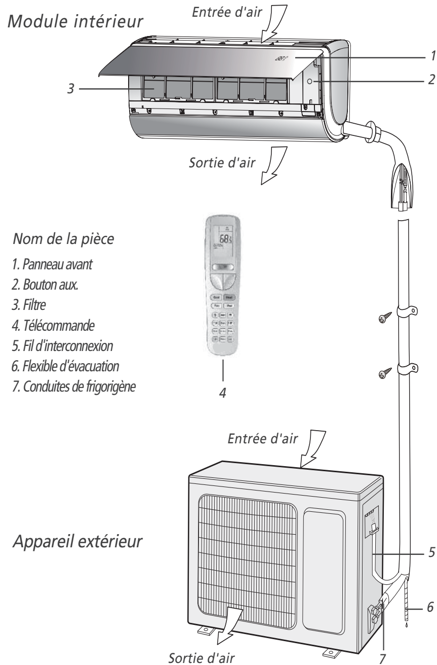
Fig. 1 - Module intérieur/Appareil extérieur
